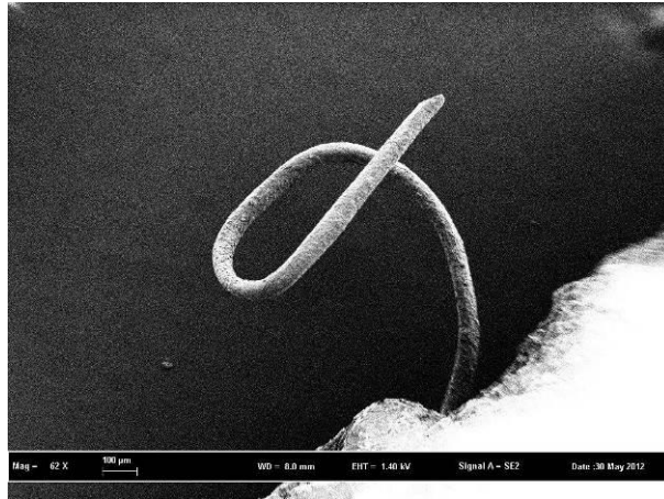
7. Image d'un cheveu prélevé dans un sceau de Carloman, examiné au microscope électronique à balayage AN, K 5, n° 11/1 – Cliché Raphaël Weil
